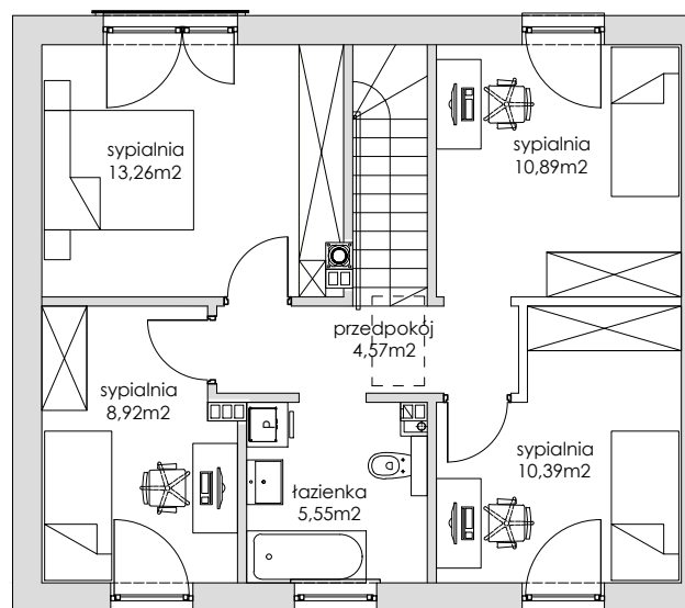
Poddasze
