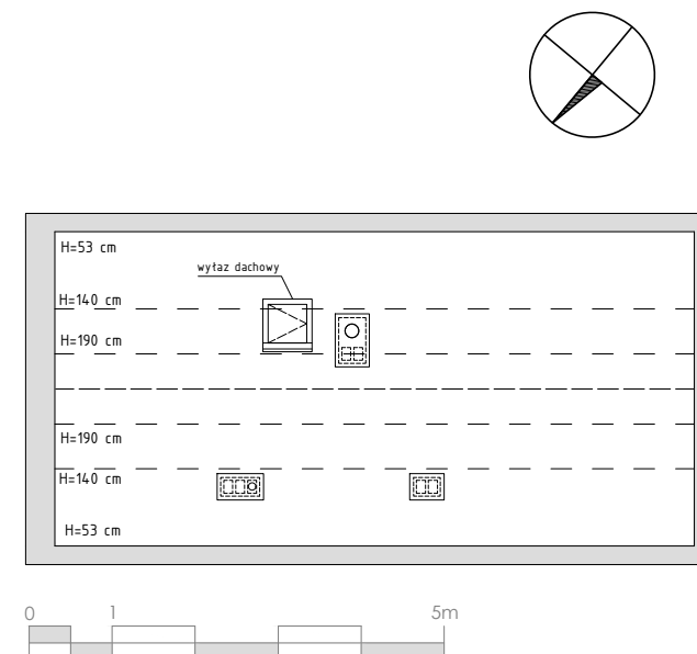
Strych
